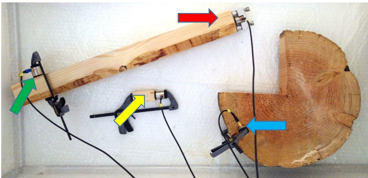
Abb. 1: Probenzusammenstellung zur Verifikation des Messaufbaus
