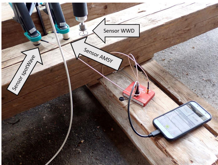
Abb. 3: Mobiles Messgerät „spotWave“; Prototyp im Test; oben im Bild links der zugehörige Sensor, in der Mitte ein gleicher Sensor, rechts der Sensor des „Woodworm Detectors“ (Foto: Jos Creemers)
