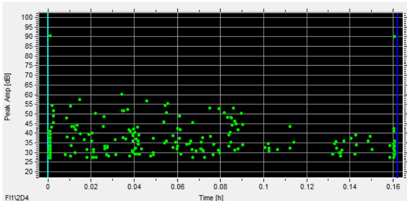
Abb. 7 oben: Messung an drei aneinandergereihte Proben zusammen, nur mittlere mit Larve besetzt; Sensor rechts an der Stirnseite einer der Leerproben
