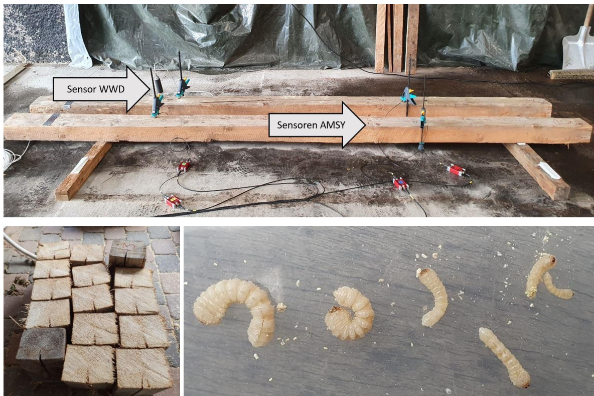
Abb. 4: oben 2 Kanthölzer mit Sensoren jeweils \frac{1}{4} Länge vom Balkenende entfernt (Fotos: U. Noldt)
